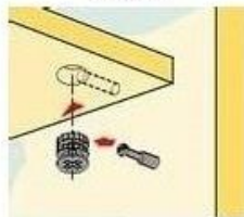
Схема установки эксцентриковой стяжки
