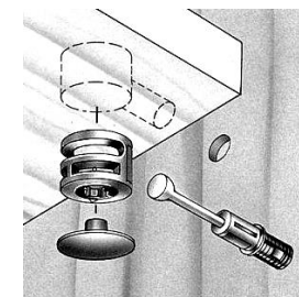
Схема установки эксцентриковой стяжки
