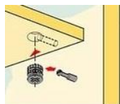
Схема установки эксцентриковой стяжки
