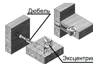
Рис.1 (Сборка деталей №3,4,7)
