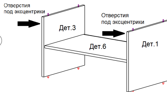
Рис.4: соединение деталей №1,3,6 (левосторонняя сборка)
