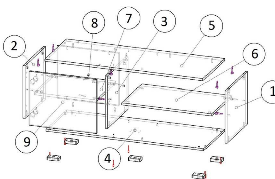
Схема установки эксцентриковой стяжки
