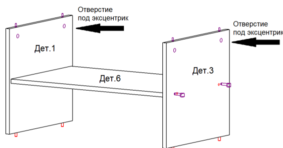
Рис.4: соединение деталей №1,3,6 (левосторонняя сборка)
